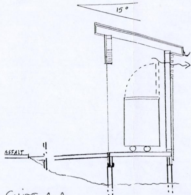
SNITT A-A
