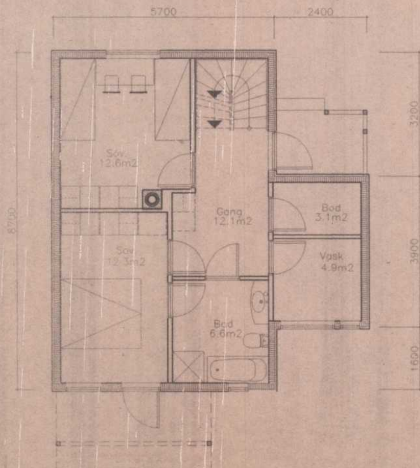
Plan 2. etasje Bruksareal = 54.0m 2
