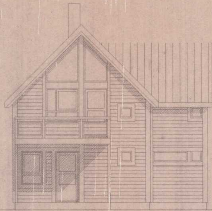
Fasade mot Sør-vest
