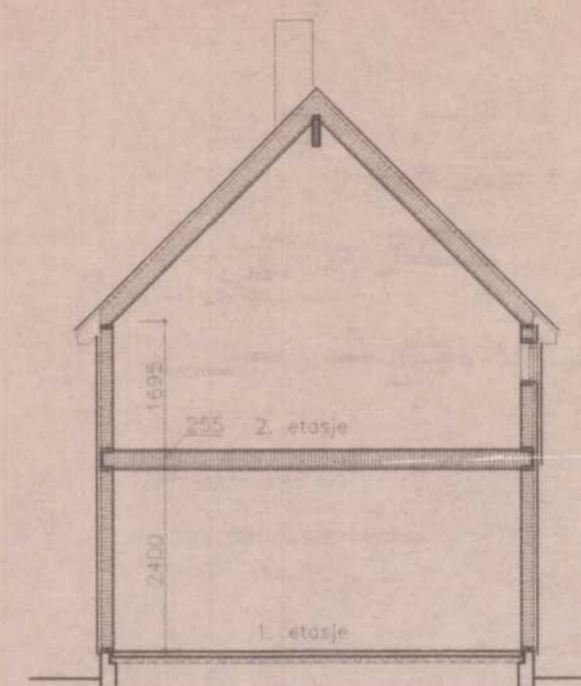
Snitt A-A
