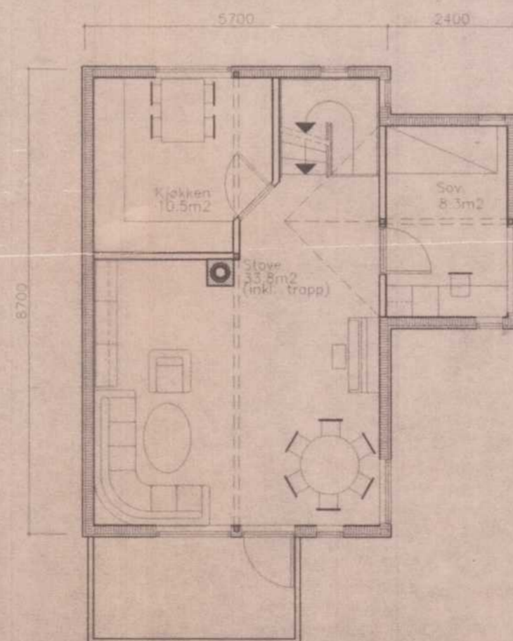
Plan 2. etasje Bruksareal = 54.0m 2
