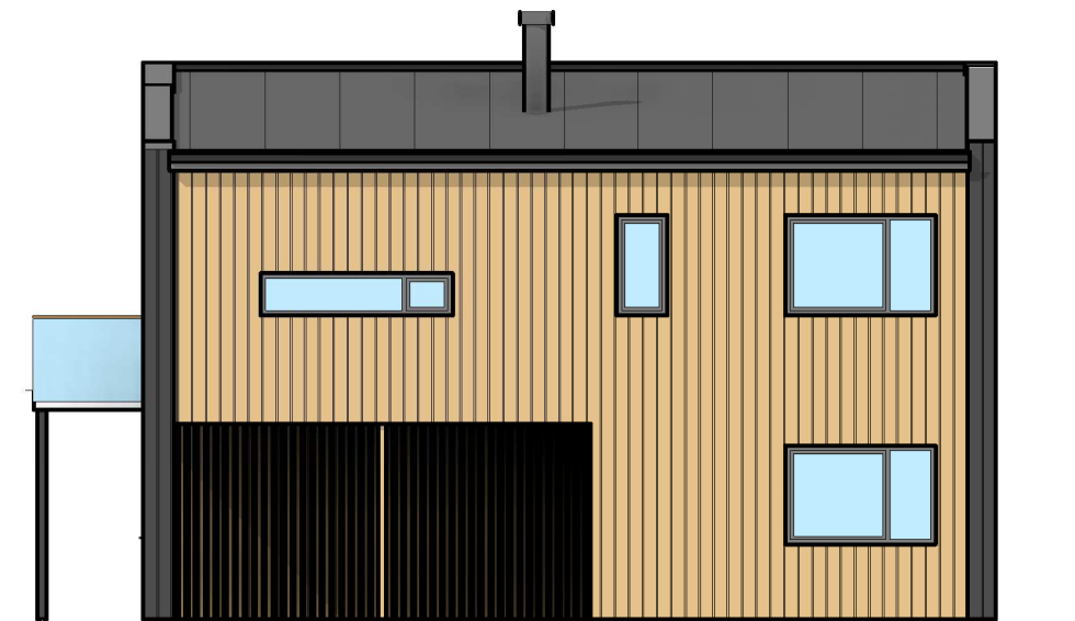
Fasade Øst 1 : 100
