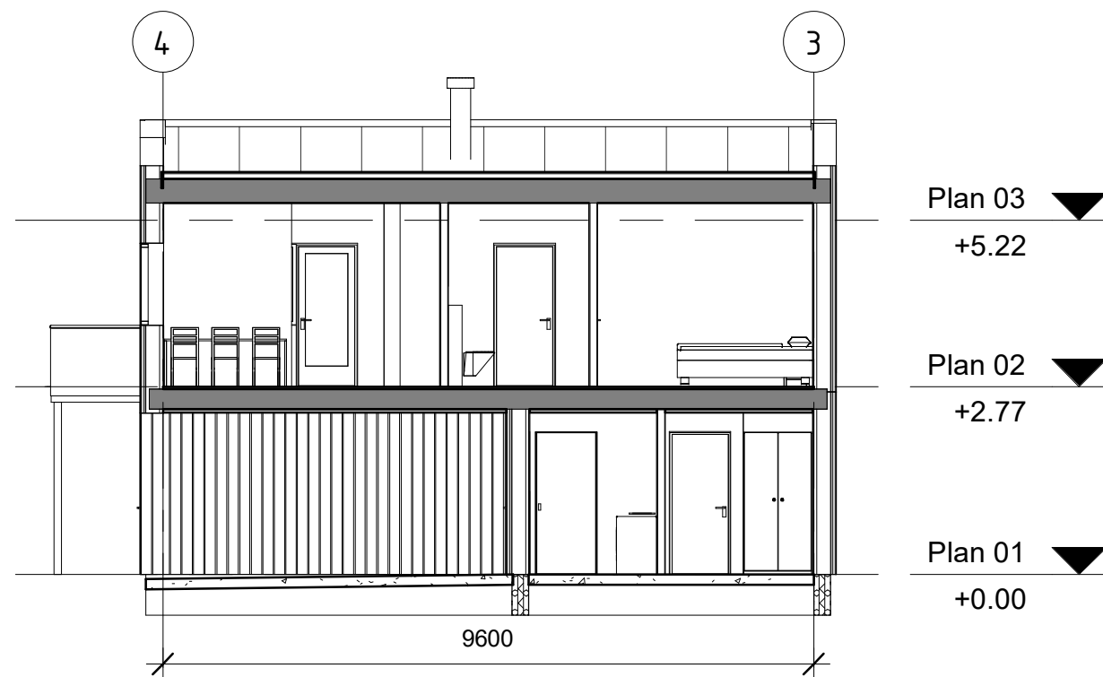
Snitt B-B 1 : 100
