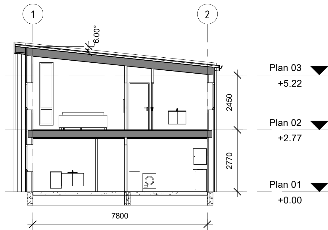
Snitt A-A 1 : 100
