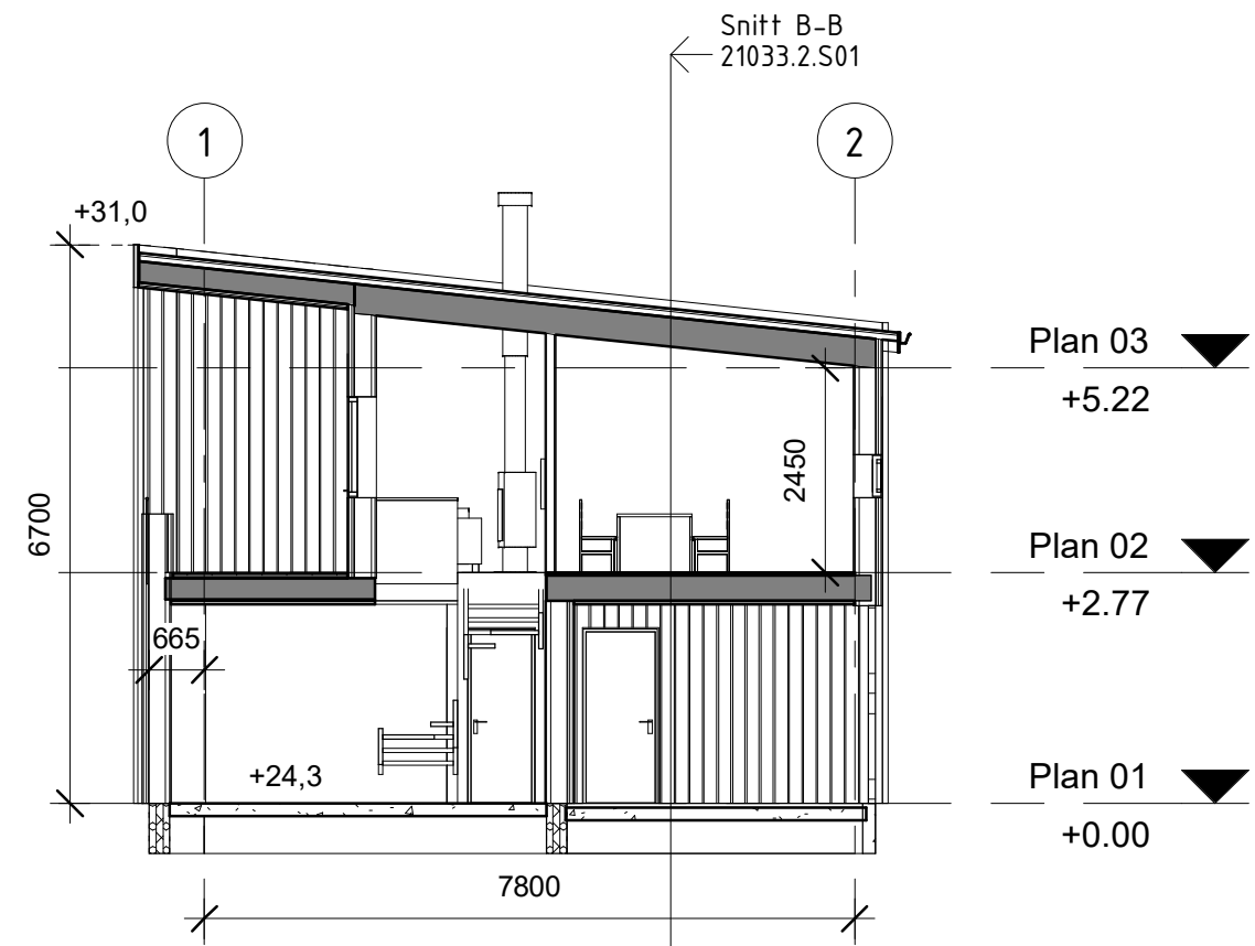
Snitt C-C 1 : 100
