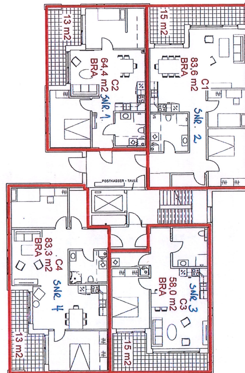
BYGG C PLAN 1 1:100
