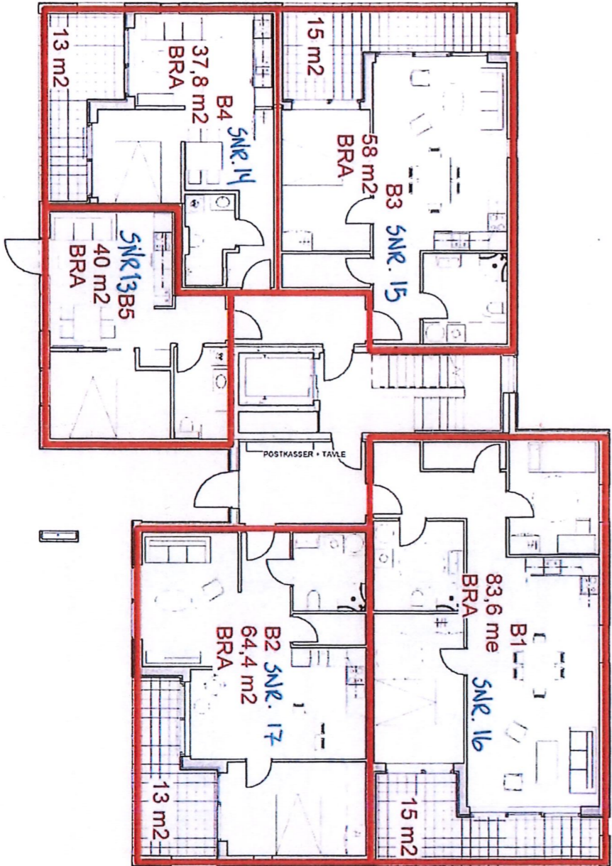
BYGG B PLAN 1 1:100
