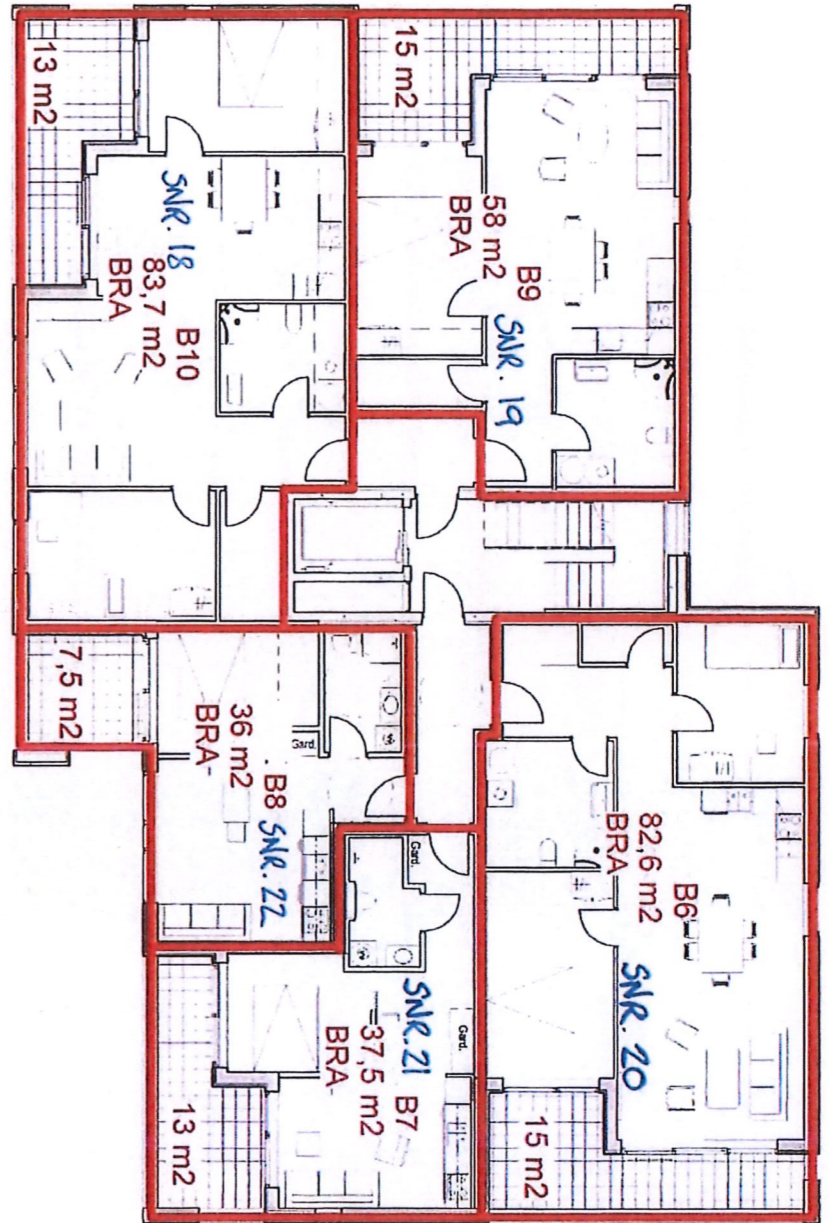
BYGG B PLAN 2 1:100
