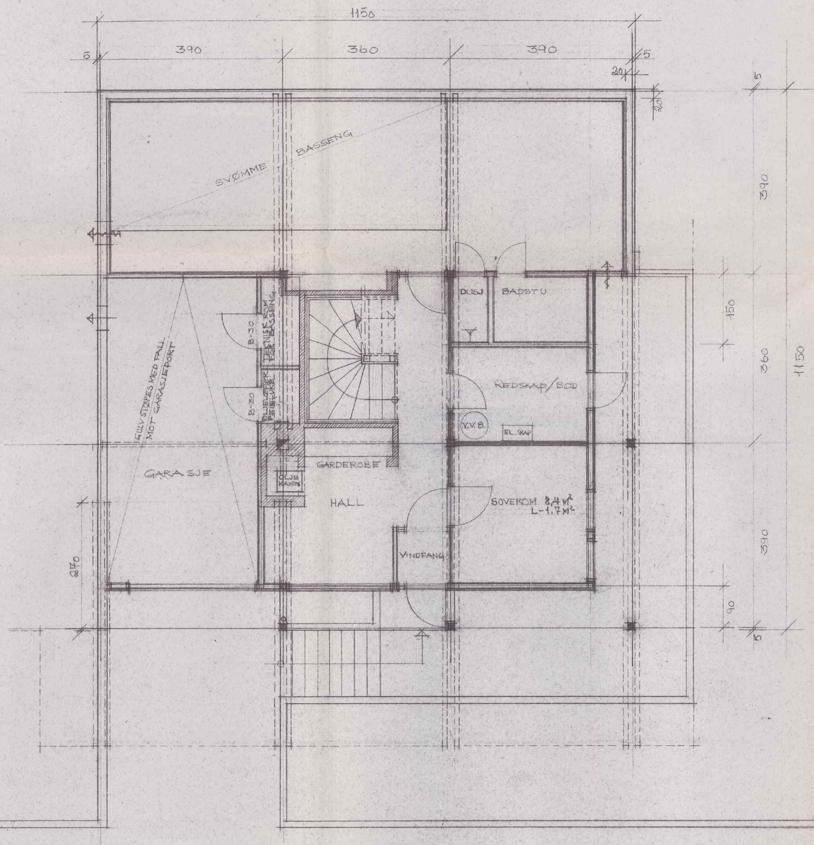
PLAN 1. ETASJE
