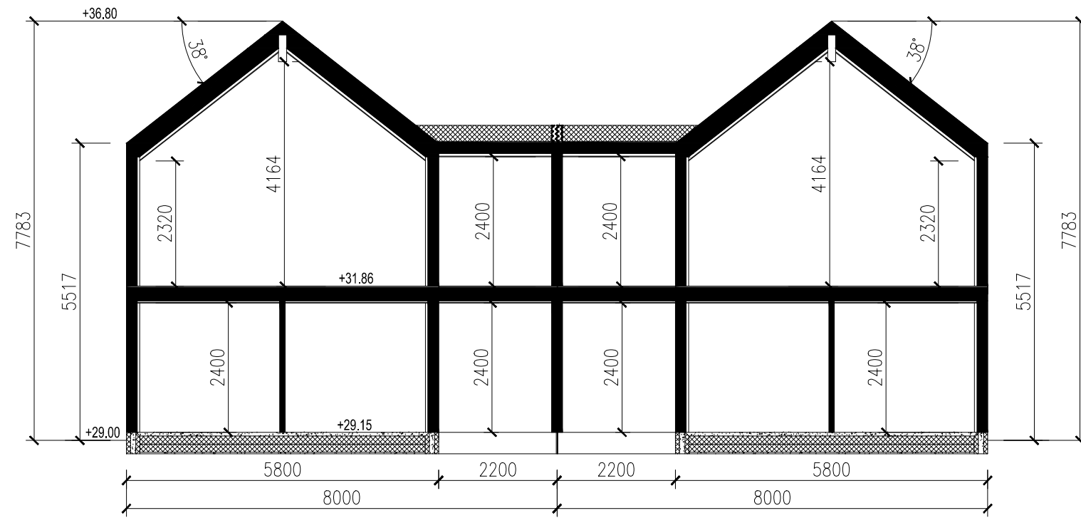
SNITT A-A
