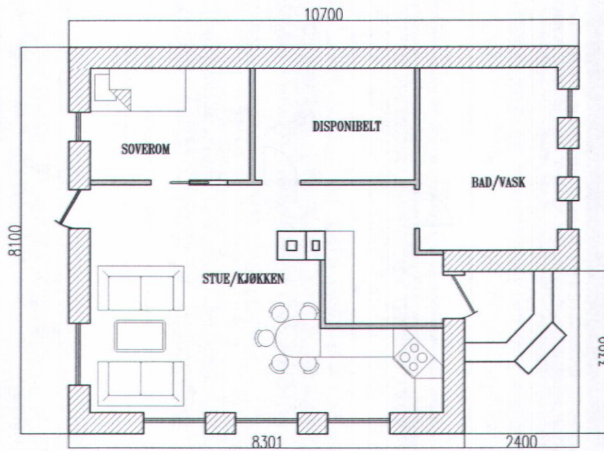
Eksisterende situasjon i underetasje
