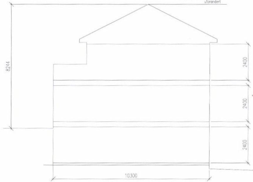
SNITT MED NYTT TRAPPEHUS
