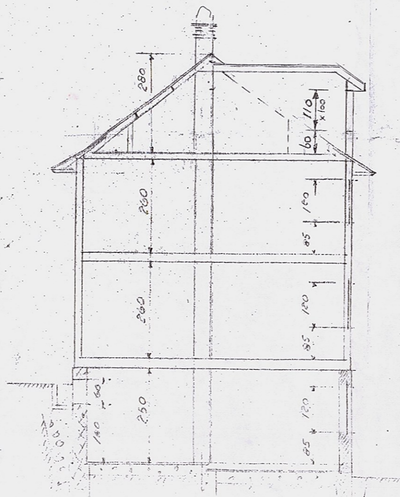
SNITT
