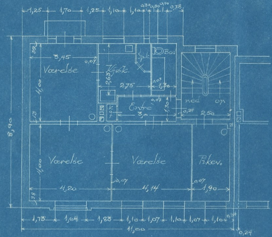
2den og 3die etasje
