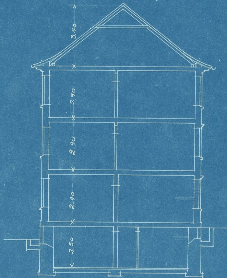
TVERSNIT.
